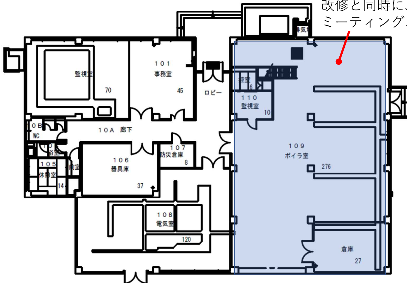
エネルギーセンター 平面図
